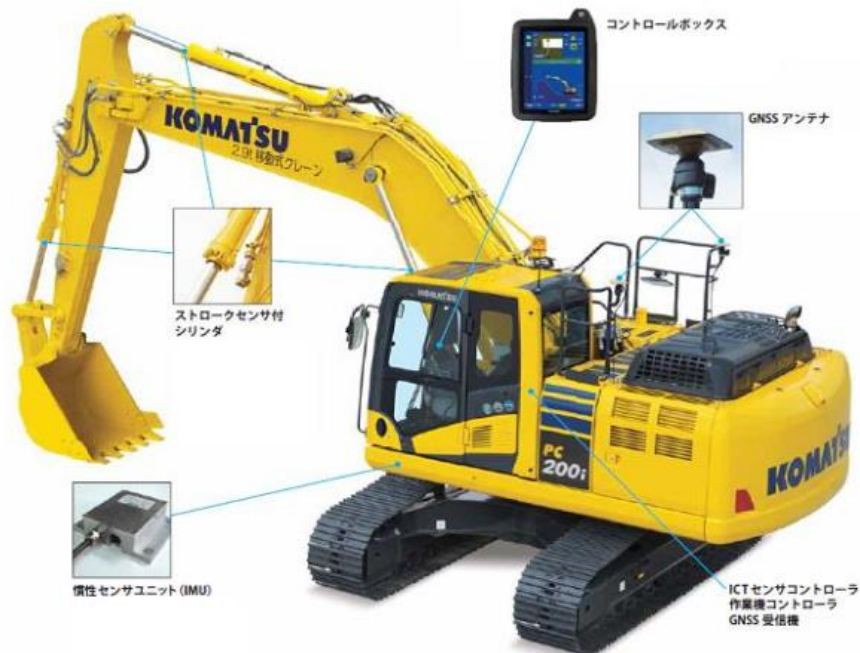
インテリジェントマシンコントロール油圧ショベル概要
